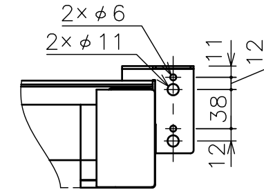
サイドブラケット詳細図 (S=1/5)
