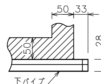
下パイプ詳細図 (S=1/5)
