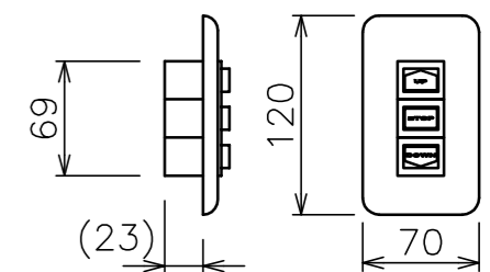
仕様：モダンプレート (ミルク-ホワイト) 一連用壁埋込スイッチ
