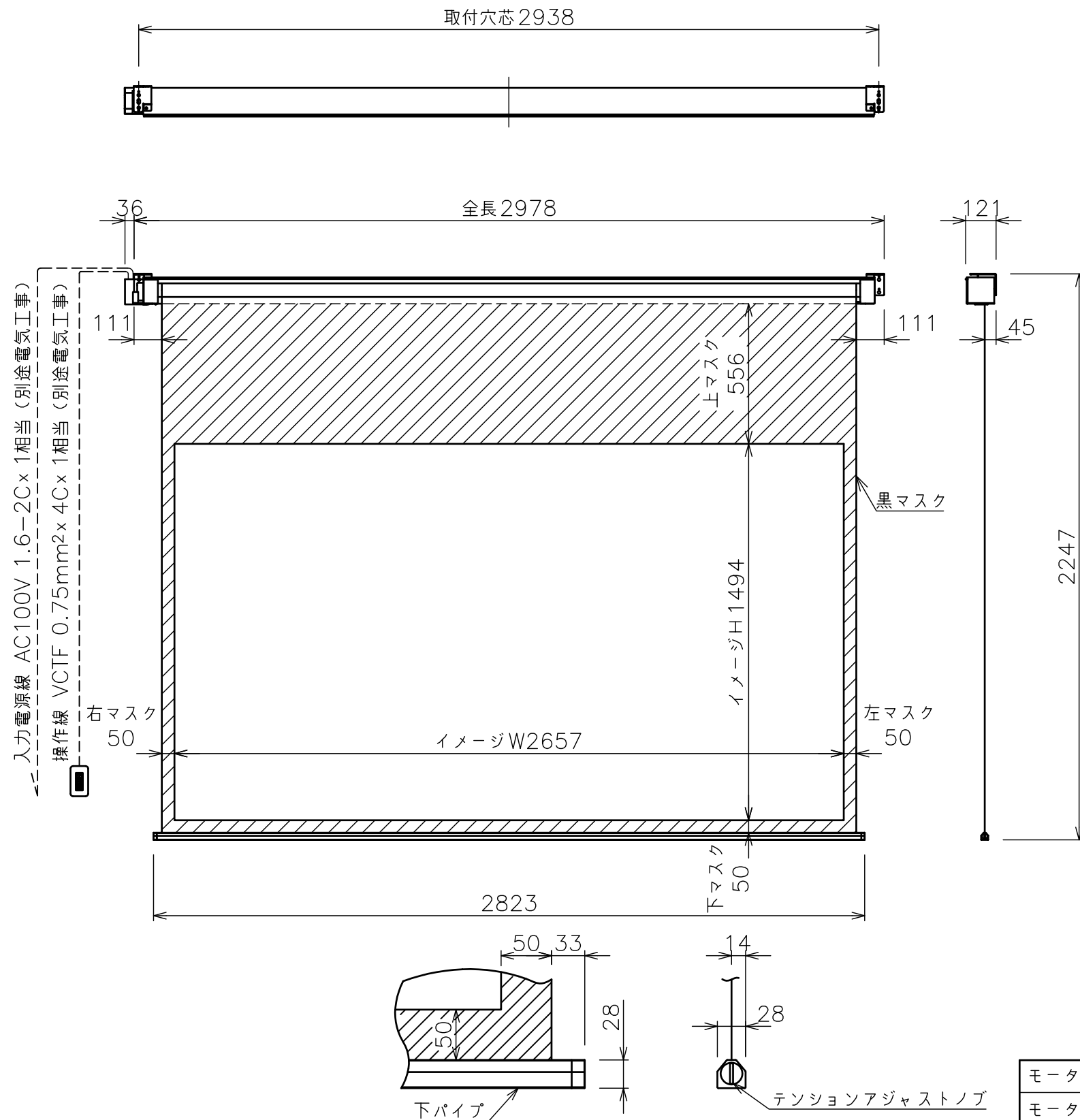
下パイプ詳細図 (S=1/5)
