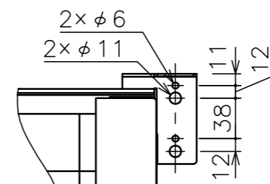
サイドブラケット詳細図 (S=1/5)
