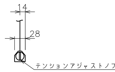
下パイプ詳細図 (S=1/5)
