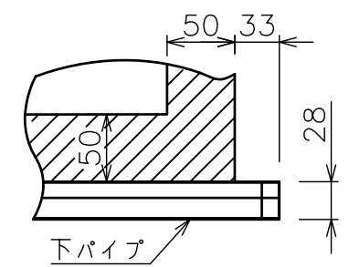
下パイプ詳細図 (S=1/5)
