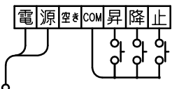
結線図
