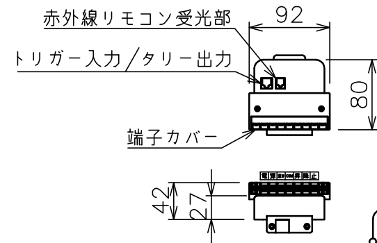
回路ボックスおよび操作スイッチ (S=1/6)
