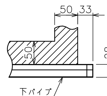
下パイプ詳細図 (S=1/5)
