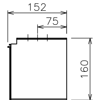
サイドブラケット詳細図 (S=1/6)
