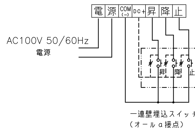
結線図
