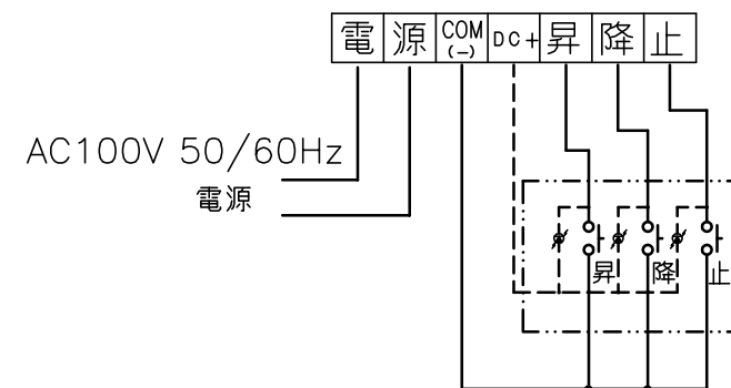
結線図
