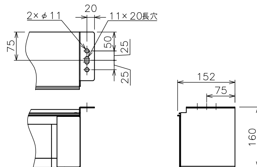
サイドブラケット詳細図 (S=1/6)
