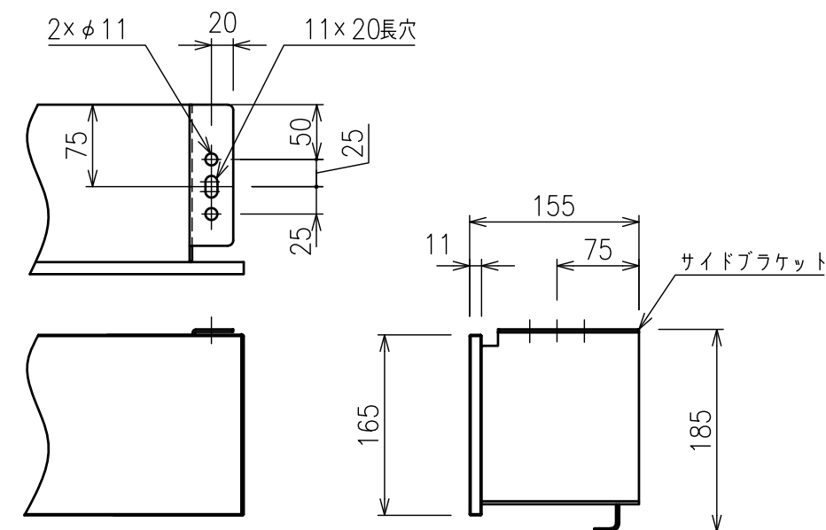
サイドブラケット詳細図(S=1/5)
