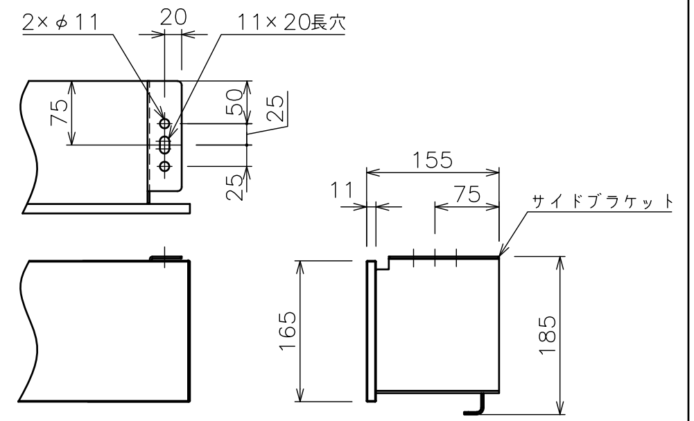
サイドブラケット詳細図(S=1/5)
