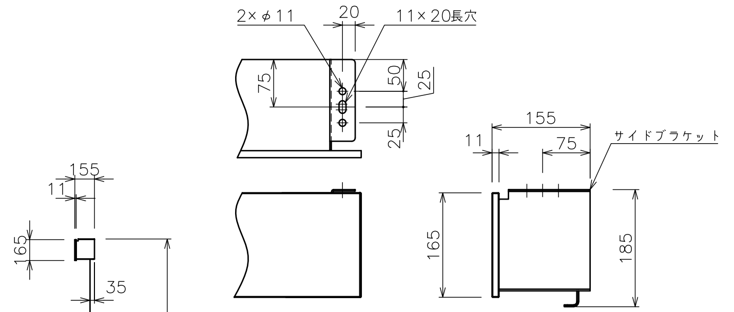
サイドブラケット詳細図(S=1/6)
