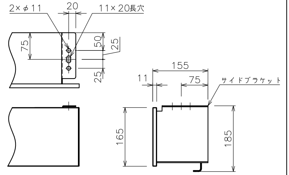
サイドブラケット詳細図(S=1/5)
