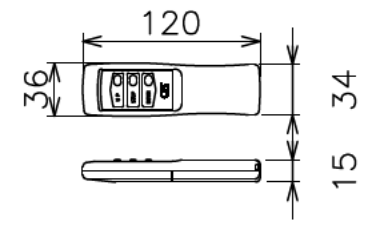
赤外線リモコン送信機/受光部
