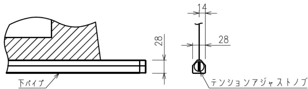
下パイプ詳細図(S=1/5)
