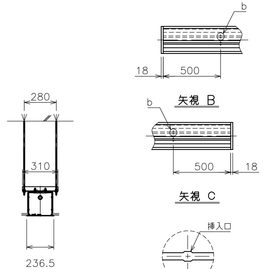
"b"部 M10ボルト挿入口拡大図
