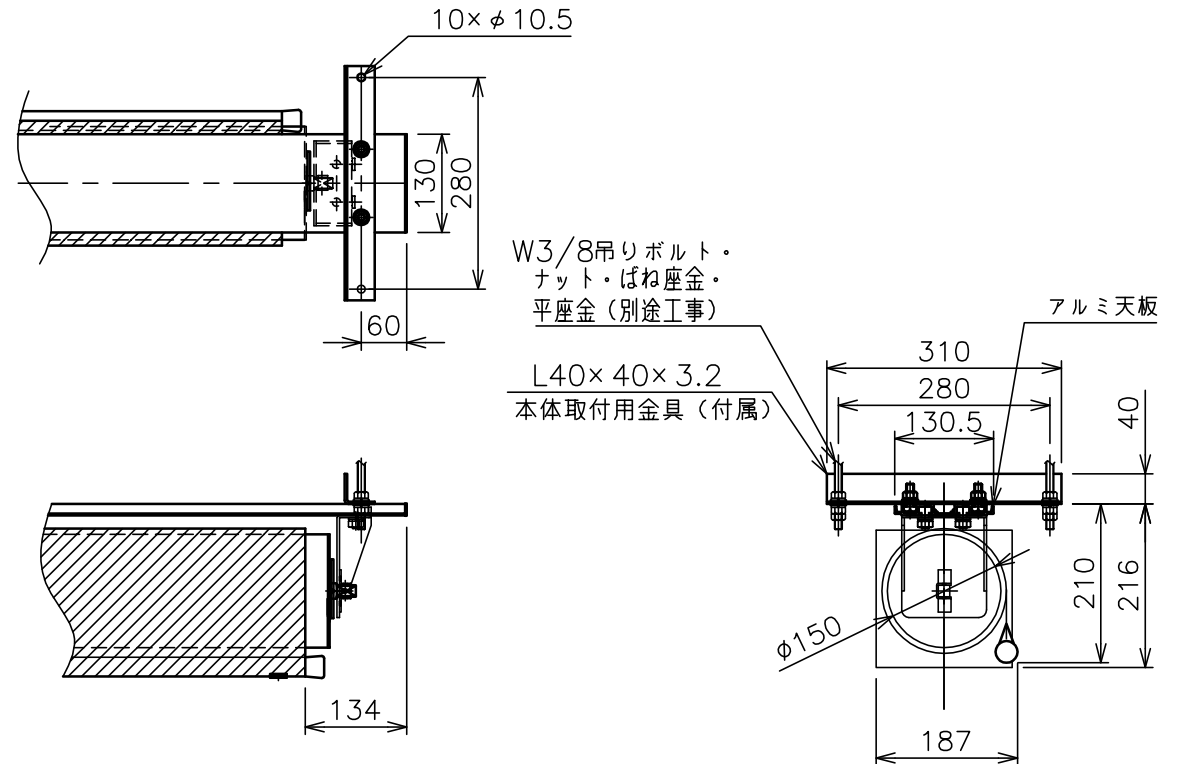
本体取付用金具詳細図 (S=1/10)
