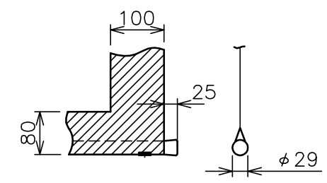
下パイプ詳細図 (S=1/10)
