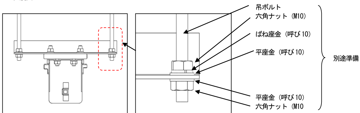
A 矢視図
