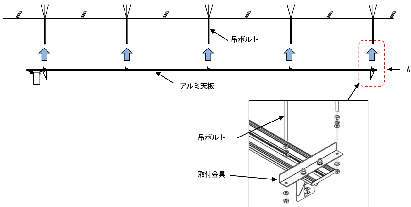
A 矢視図
