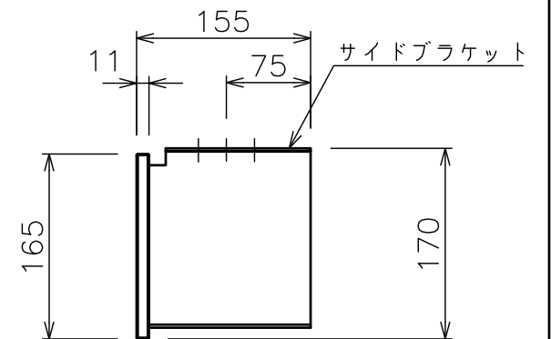
サイドブラケット詳細図 (S=1/6)
