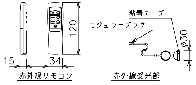
回路ボックスおよび操作スイッチ (S=1/8)
