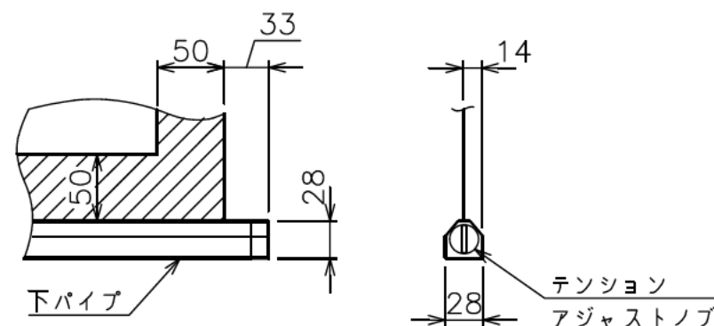
下パイプ詳細図 (S=1/5)
