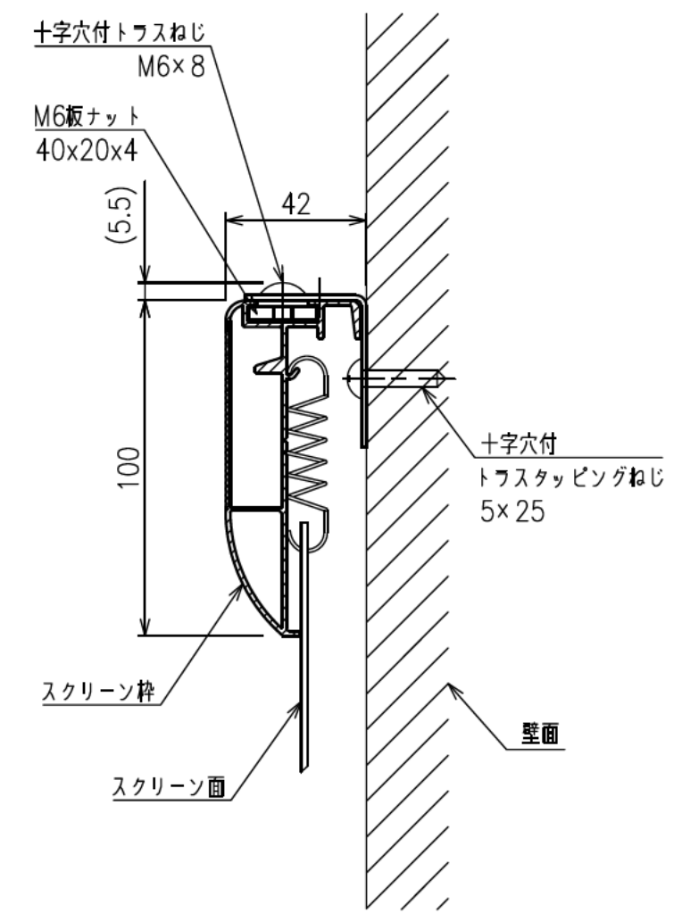
A-A断面拡大図
