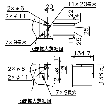
サイドブラケット (S=1/8)
