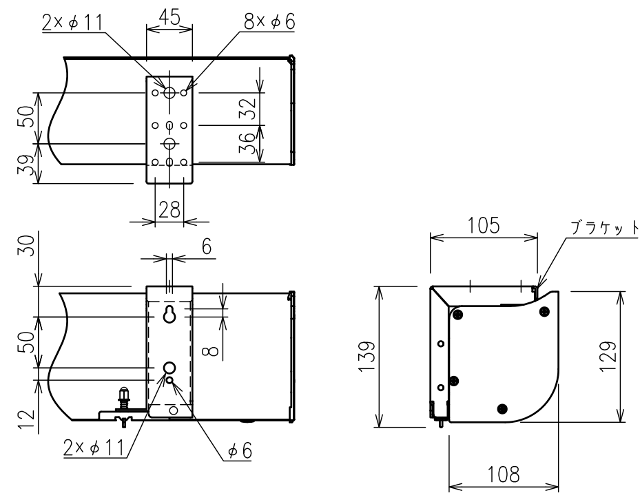
a部詳細
