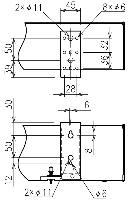
α部詳細
