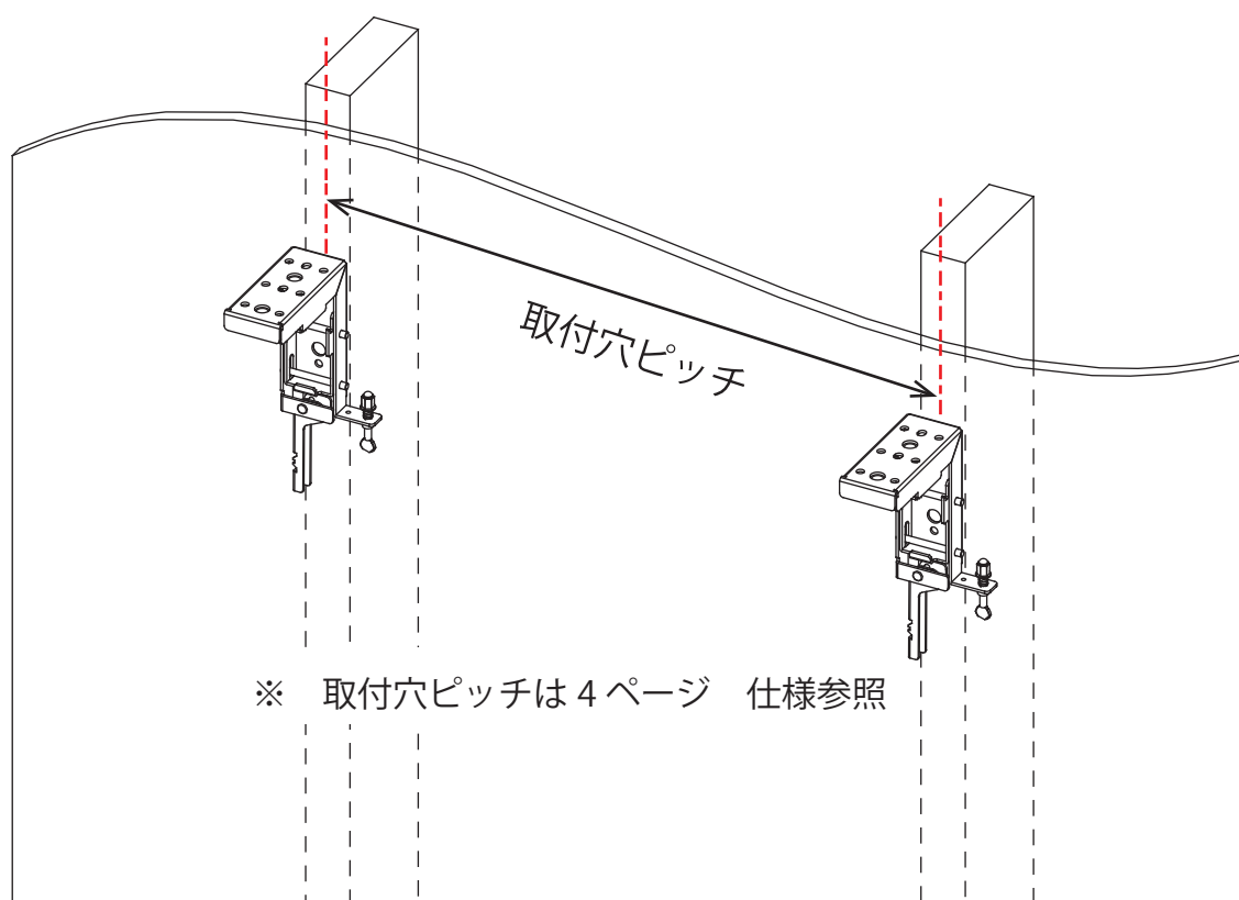
壁面取付例
