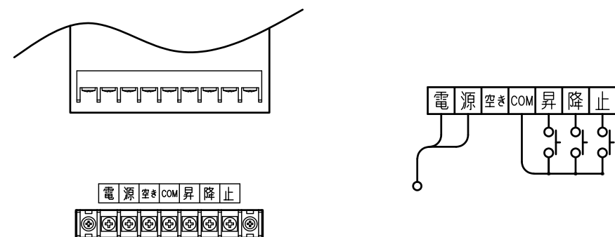
接続詳細
