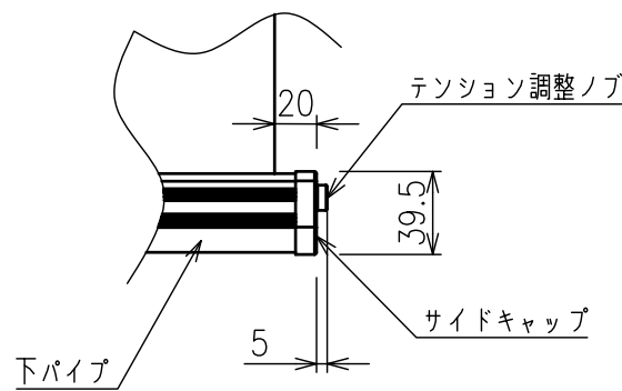
b 部詳細
