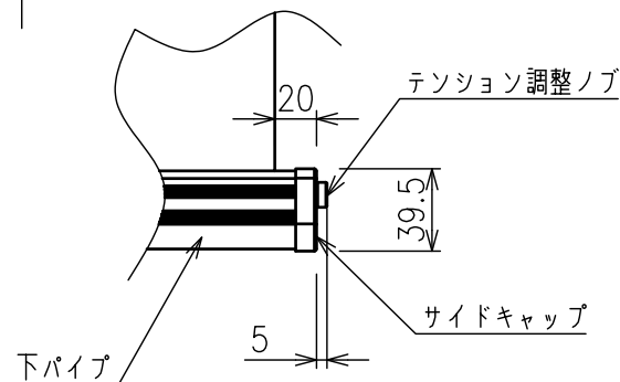
b 部詳細
