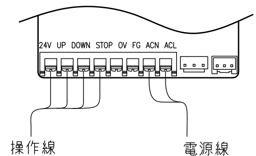
接続詳細
