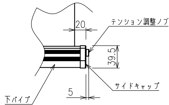
b 部詳細
