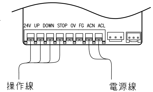
接続詳細
