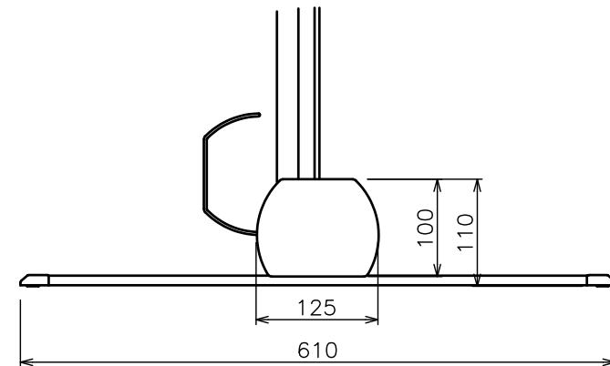
a部拡大図 (S=1/5)
